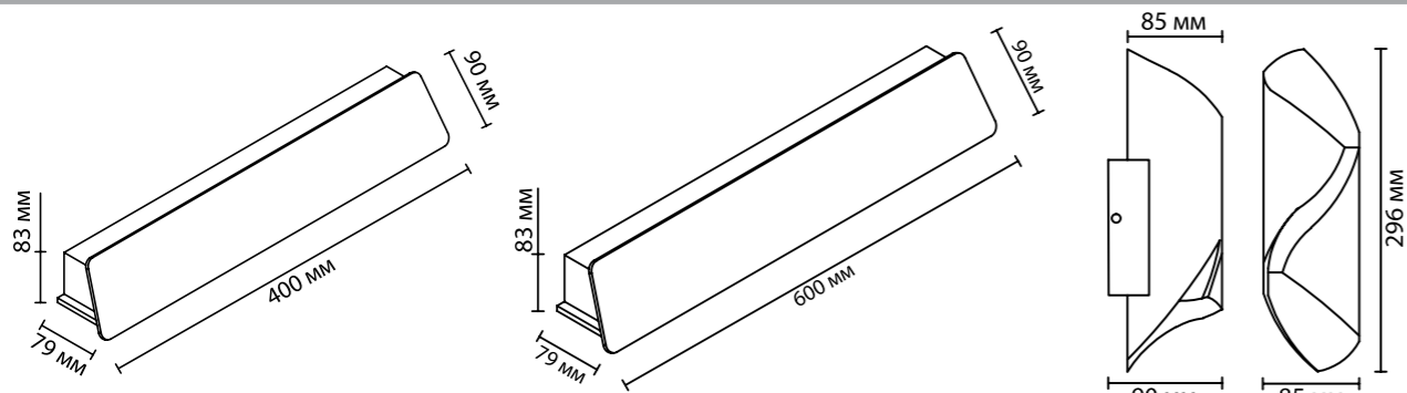
6642/12WL 1×LED×12W, 1083 lm крепёж: планка
