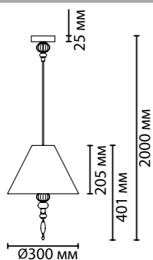
4896/1 1 × E27 × 40W крепеж: планка
