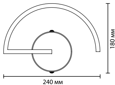
4308/8WL 1 × LED × 8W, 480 lm крепёж: планка
