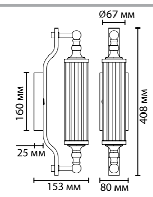
4941/1W, 4942/1W, 4943/1W 1 × E14 × 40W крепеж: планка, выкл. на базе
