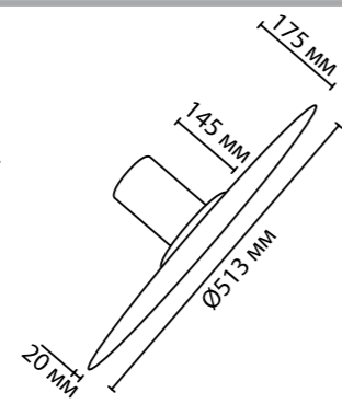
5078/45L 1×LED×45W крепеж: планка
