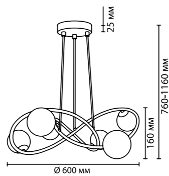
4807/6 6 × G9 × 40W крепеж: планка
