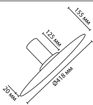
5078/35L 1×LED×35W крепеж: планка
