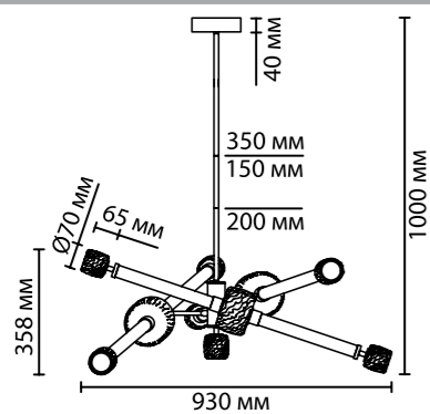
5426/54CL, 5427/54CL 1×LED×54W, 3515 lm крепёж: планка
