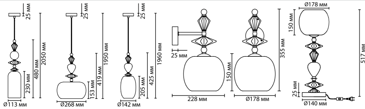
4855/1 1 × E14 × 40W крепеж: планка
