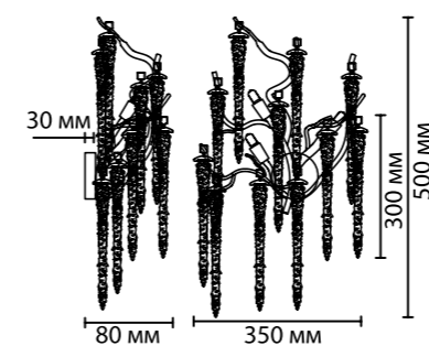
5005/3W 3 × G9 × 40W крепеж: планка
