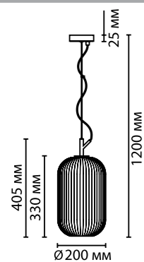
4751/1 1 × E27 × 60W крепеж: планка
