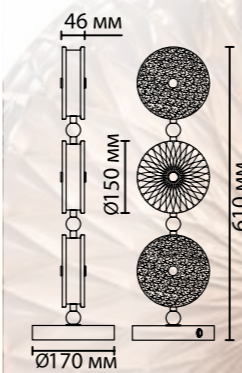
5412/13TL 1 × LED × 18W, 950 lm выкл. на основании
