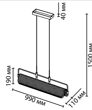
5055/35L, 5055/35LA 1 x GU10 LED x 35W, 2584/ 2548 lm крепёж: планка
