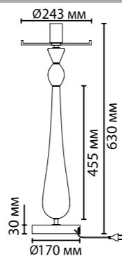
4868/1T, 4889/1T 1 × E27 × 60W, база выкл. на основании
