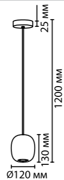
5053/1A, 5053/1B, 5053/1C 5053/1G 1 × GU10 × 4W крепёж: планка
