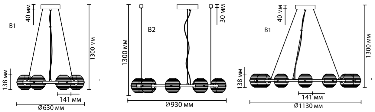
5041/60L 1×LED×60W, 6086 lm крепеж: планка 5041/90L 1×LED×90W, 7751 lm крепеж: планка 5041/120L 1×LED×120W, 9363 lm крепеж: планка
