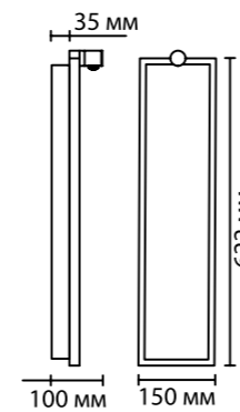
5078/30WL 1×LED×30W крепеж: планка
