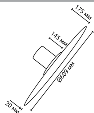
5078/55L 1×LED×55W крепеж: планка
