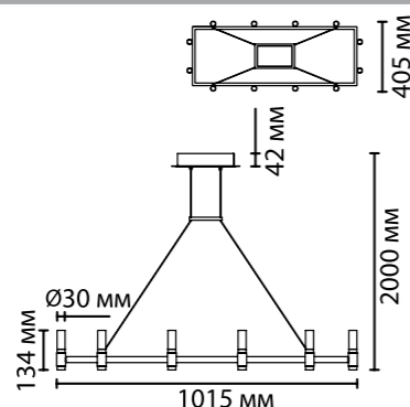
5009/48LA 1 × LED × 48W, 1900 lm крепёж: планка
