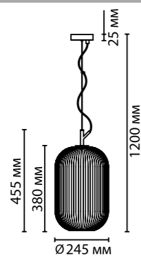
4752/1 1 × E27 × 60W крепеж: планка
