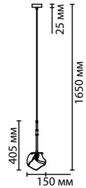
4789/1 1 × G9 × 40W крепеж: планка
