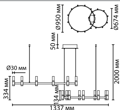
5009/98LA 1 × LED × 98W, 3300 lm крепёж: планка
