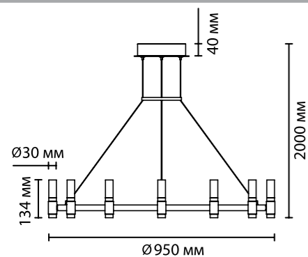
5009/48L 1 × LED × 48W, 1900 lm крепёж: планка
