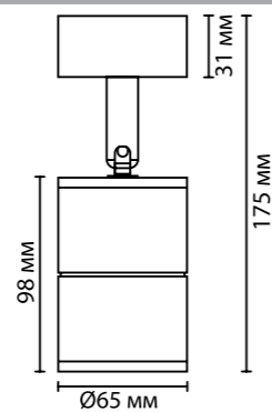
4207/1C 1×LED GU10 × 10W крепеж: планка
