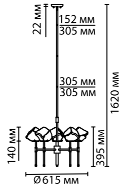
4789/5 5 × G9 × 40W крепеж: планка
