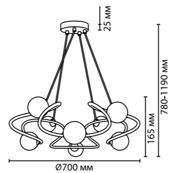
4806/8 8 × G9 × 40W крепеж: планка
