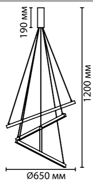
3860/48L 1 × LED × 48W, 2700 lm крепёж: планка
