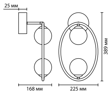
4807/2W, 4808/2W 2 × G9 × 40W крепеж: планка
