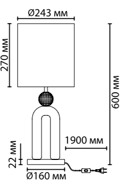
5410/1T 1 × E27 × 60W выкл. на шнуре
