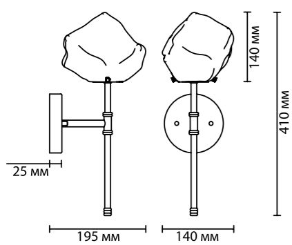
4789/1W 1 × G9 × 40W крепеж: планка
