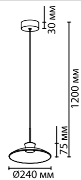
5055/9L, 5055/9LA 1 x GU10 LED x 9W, 720/ 708 lm крепёж: планка
