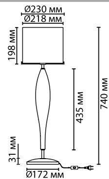
4850/1T 1 × E27 × 60W выкл. на шнуре
