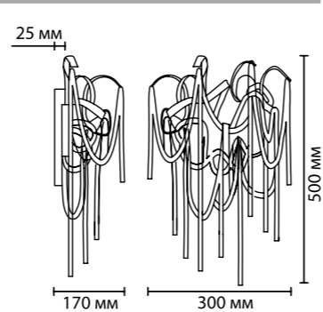
5067/4W 4 x G9 x 40W крепёж: планка
