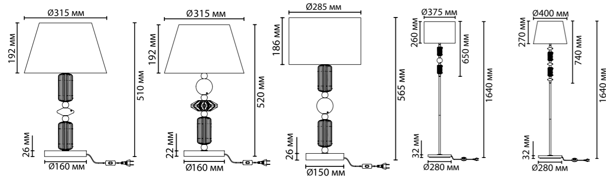
4861/1TA, 4861/1TC 1×E27×60W выкл. на шнуре
