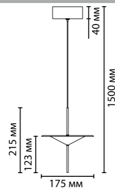
5012/10L 1 × LED × 10W, 600 lm крепеж: планка
