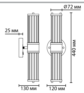
4944/2W, 4945/2W, 4946/2W 2 × E14 × 40W крепеж: планка, выкл. на базе
