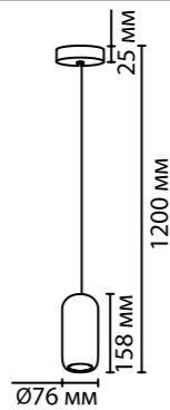
5053/1, 5053/1D, 5053/1E 1 × GU10 × 4W крепёж: планка
