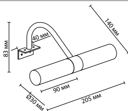
2452/2 2 × G9 × 40W крепёж: планка
